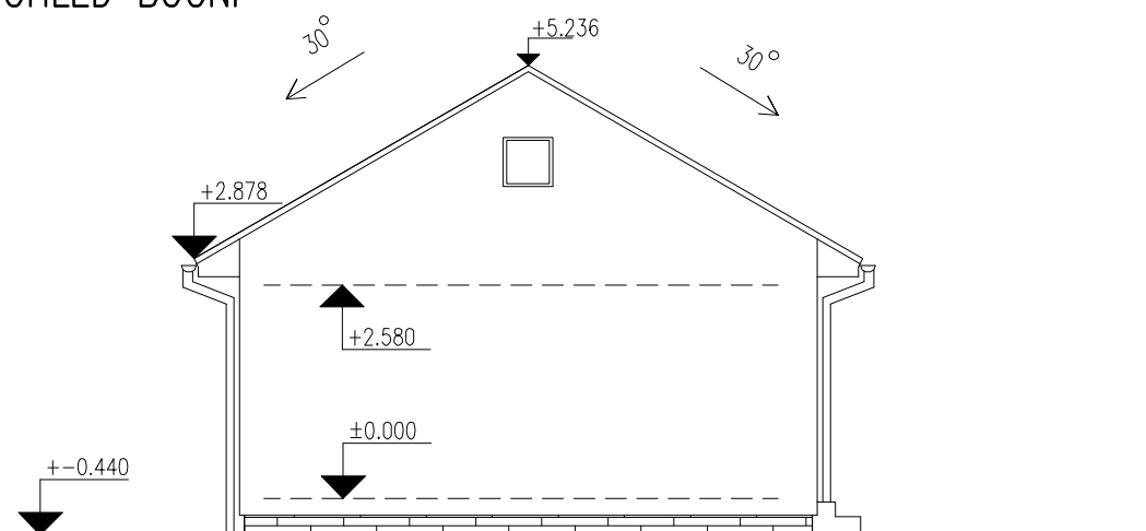
POHLED BOČNÍ
